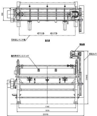
■ 特1720型 高速裁断機
