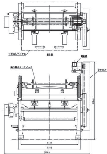
■ 特RL型 高速裁断機
