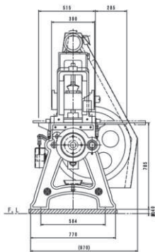
■ L型 高速裁断機
