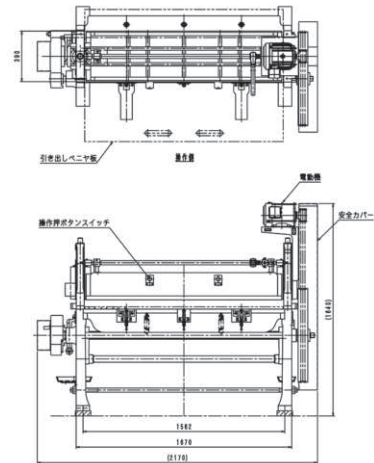
■ 特RL型 高速裁断機
